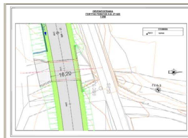
Κάτοψη γέφυρας
