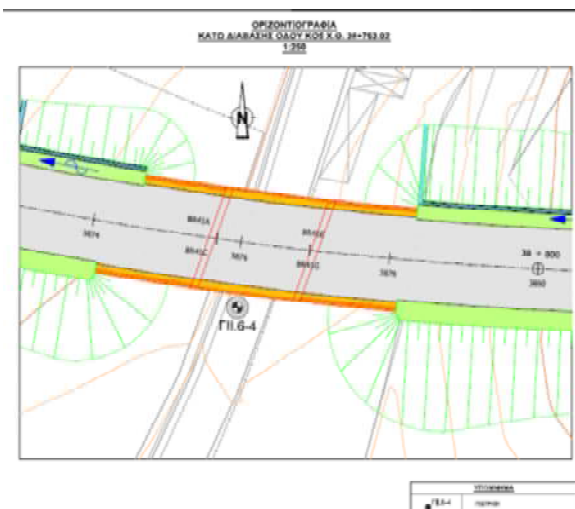
Κάτοψη κάτω διάβασης
