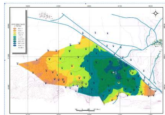
Γεωλογικός χάρτης – αθροιστικό πάχος λιγνίτη
