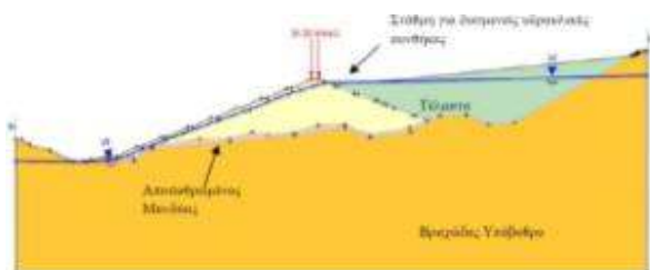
Γεωτεχνικό μοντέλο προσομοίωσης
