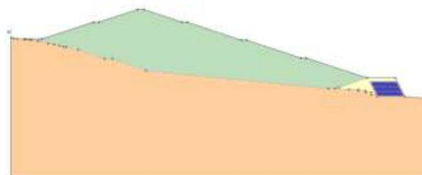
Γεωτεχνικό μοντέλο προσομοίωσης των πρηνών του τοίχου οπλισμένου γης της εσωτερικής οδοποιίας
