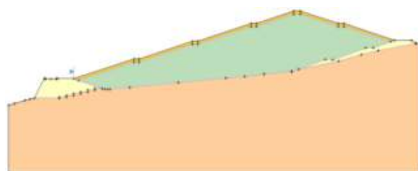
Γεωτεχνικό μοντέλο προσομοίωσης των πρηνών του απορριμματικού αναγλύφου
