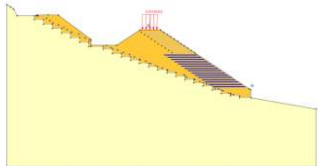
Γεωτεχνικό μοντέλο προσομοίωσης των πρανών του οπλισμένου επικώματος της εσωτερικής οδοποιίας
