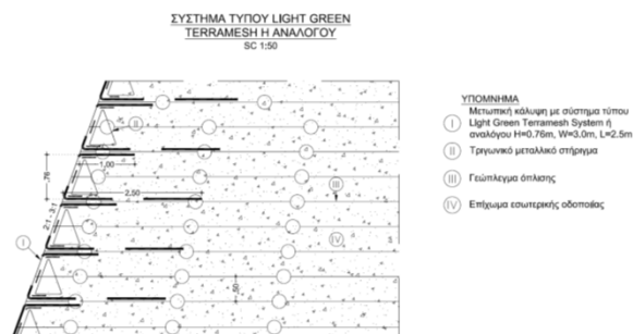
Λεπτομέρεια τοίχου οπλισμένης γης
