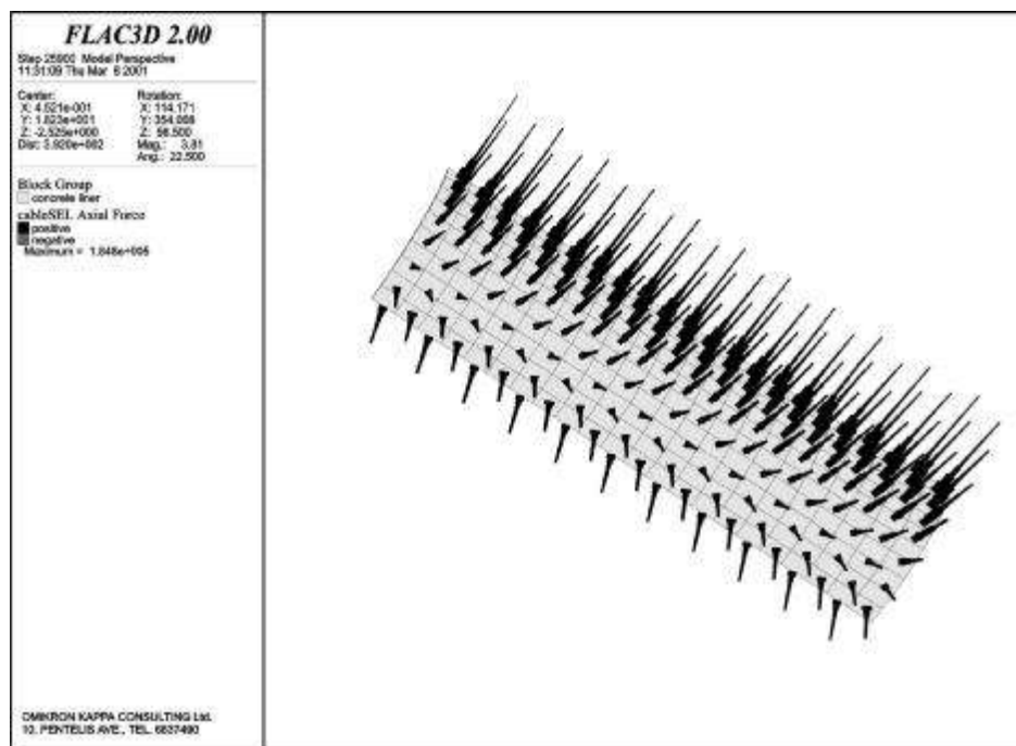
Σχήμα 8 Αξονικές δυνάμεις στα αγκύρια κατά μήκος της σήραγγας μετά το τέλος της α' φάσης εκσκαφής σε πεσοσειδή διάταξη. Κατηγορία III, K=0,9.
