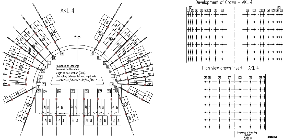
Σχήμα 4 Πρόγραμμα εκτέλεσης τσιμεντενέσεων σταθεροποίησης βραχώδους, κατηγορία IV
